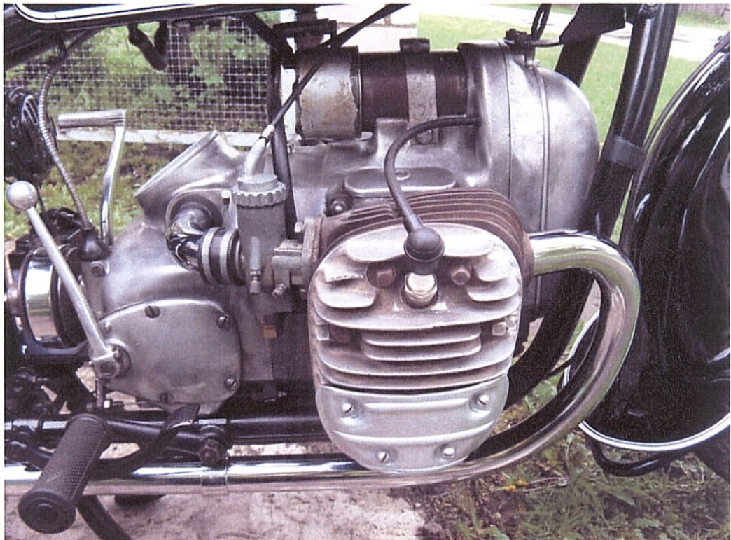
Vaade mootorile teiselt küljelt
